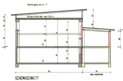
SCHEMASCHNITT
